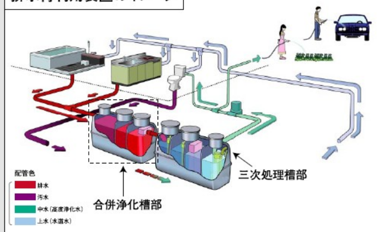
排水再利用装置のイメージ
